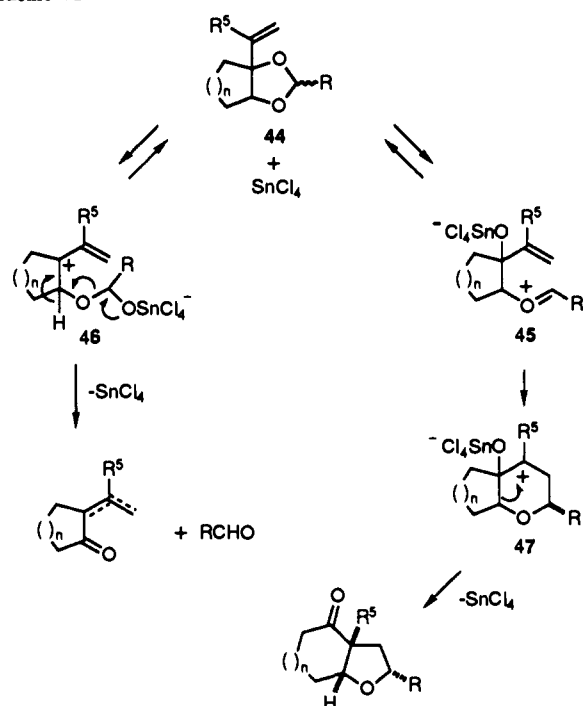
Scheme VI
